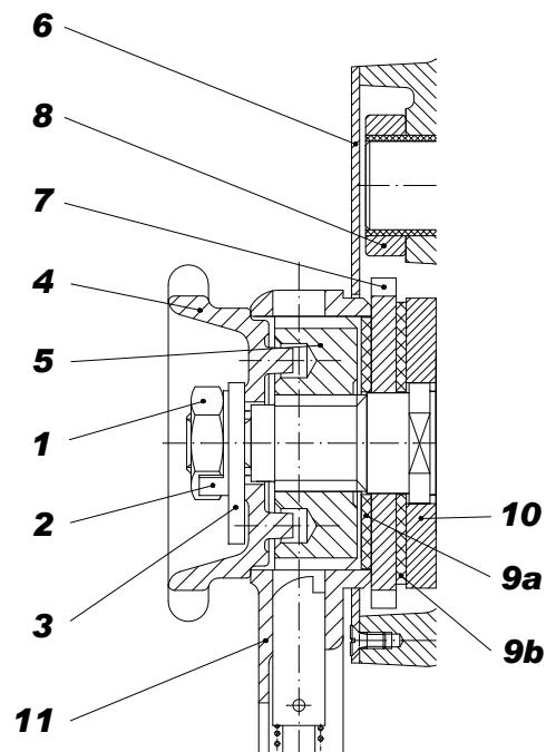
Obr. 11.3 - Montáž brzdy
